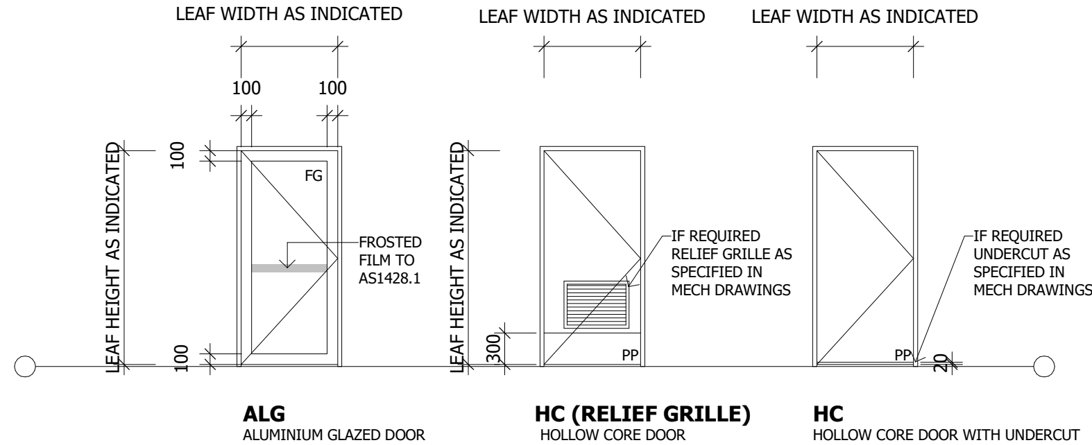
1 DOOR TYPE ELEVATIONS 1 : 50
